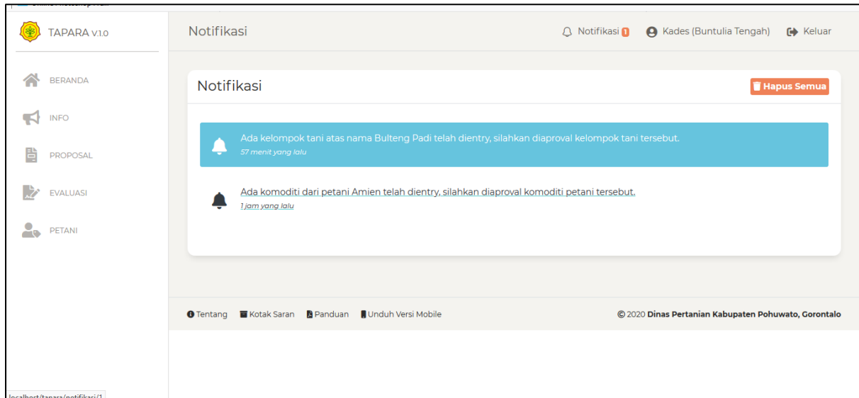
Gambar 4.1. Halaman Notifikasi
