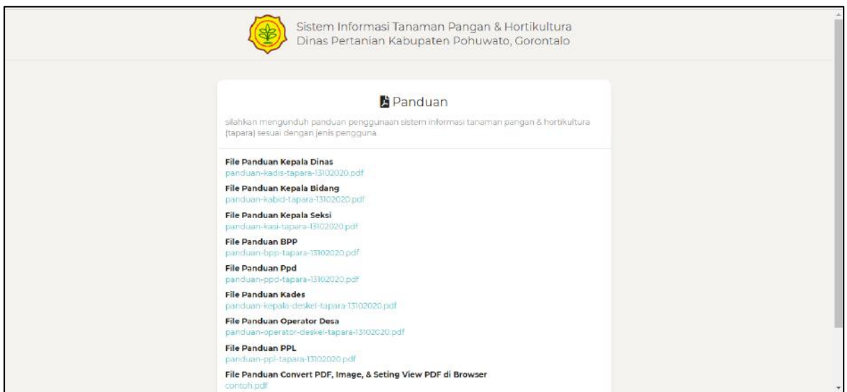
Gambar 1.4. Halaman Panduan
