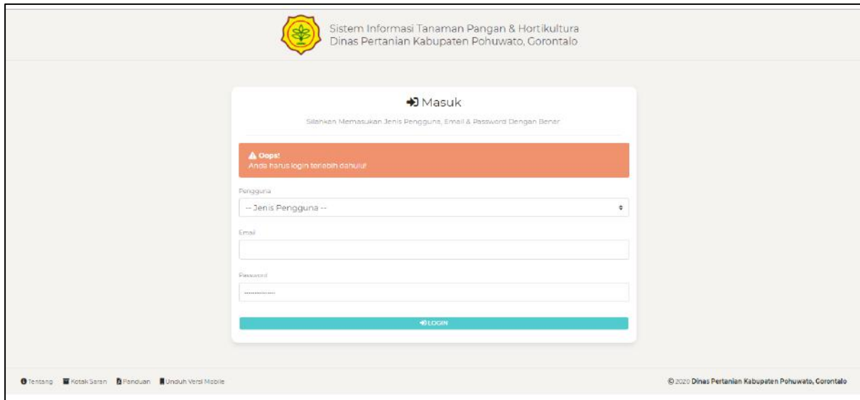
Gambar 1.1. Halaman Masuk
